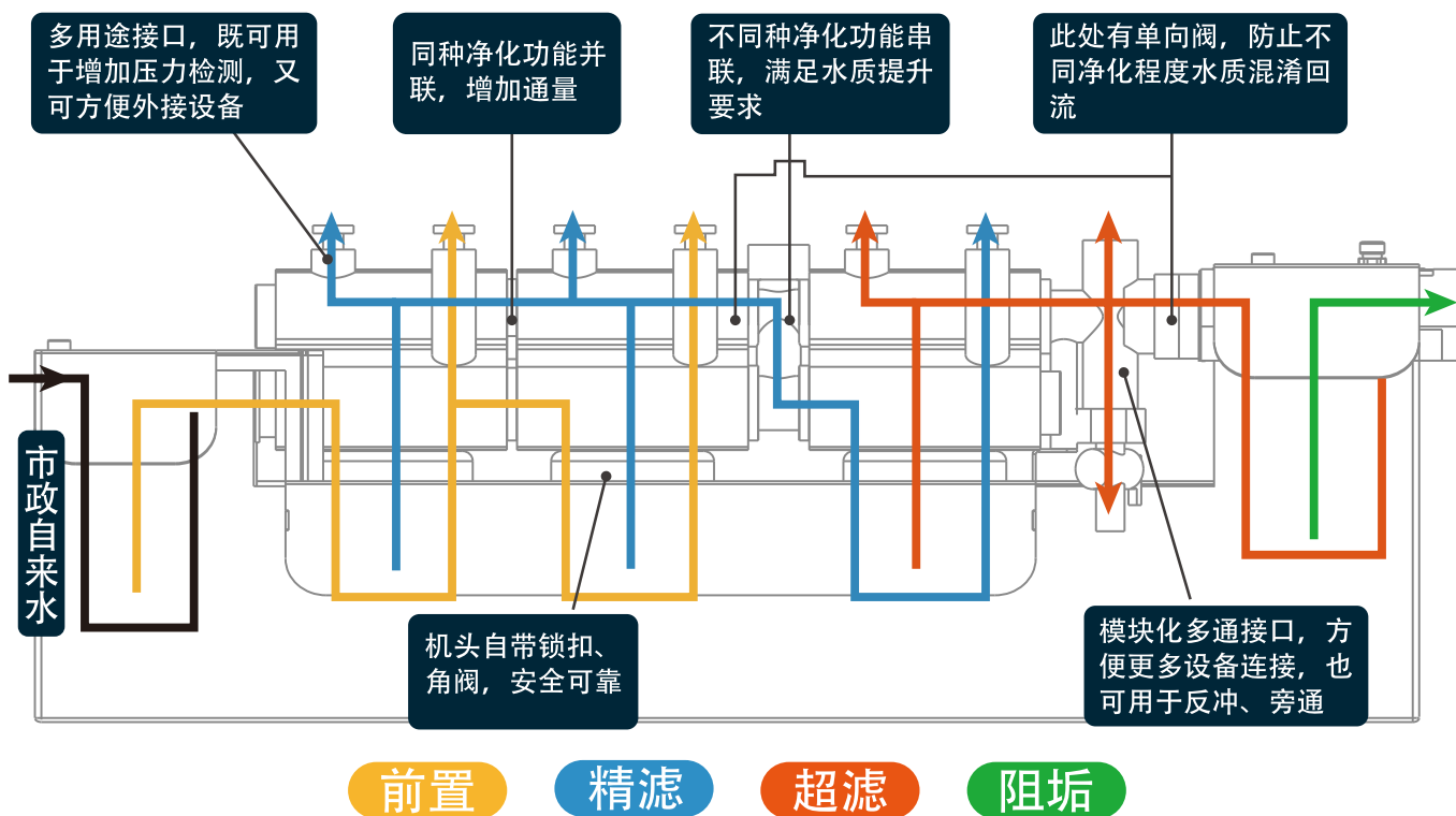
前置+并联精滤+串联超滤+阻垢
